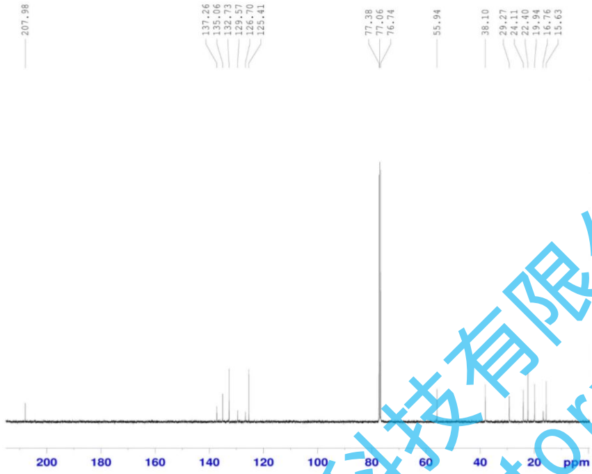
附 13 C-NMR 圖
