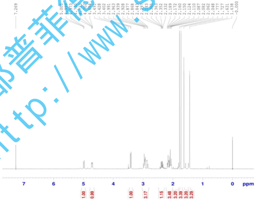
附 1 H-NMR 圖
